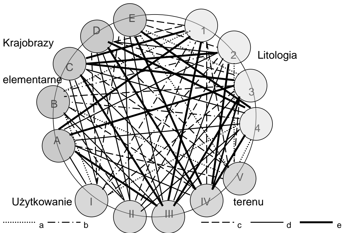
Rysunek 2. Schemat oceny stabilności krajobrazu regionu
